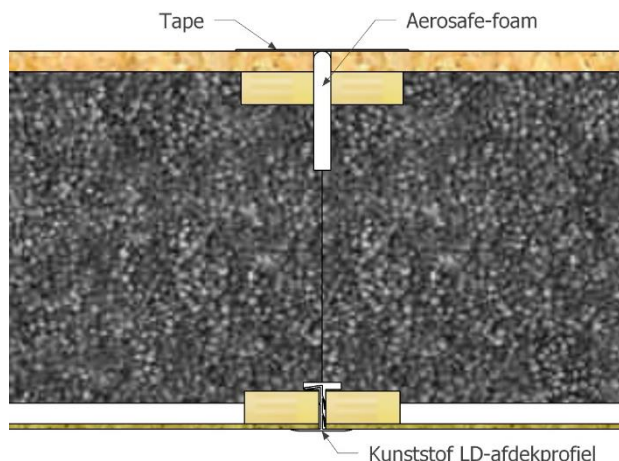
Figuur 5 - Detail verticale aansluiting
