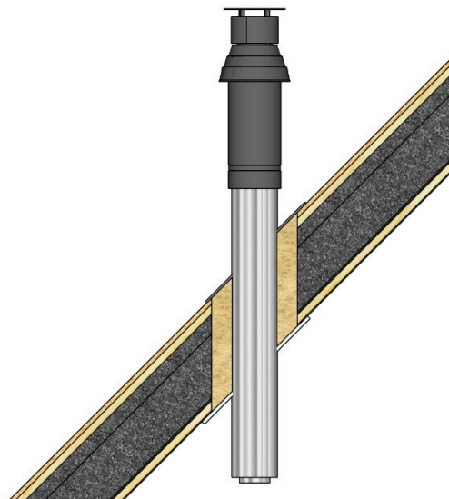
Figuur 7 - Detail sparing mantelbuis
