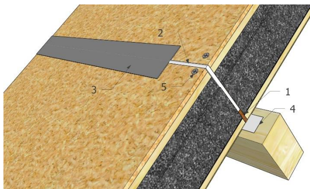
Figuur 6 - Detail horizontale naden
