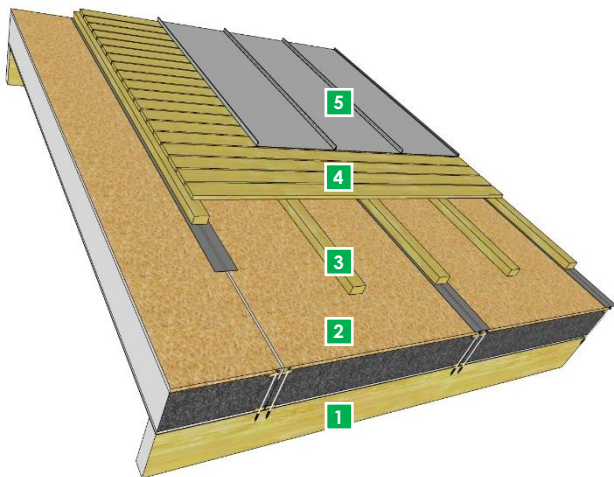
Figuur 8 - Geventileerde constructie
