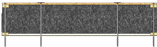
Figuur 3 - Detail bevestiging t.p.v. muurplaat
