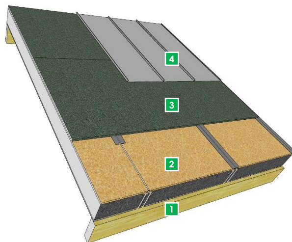
Figuur 10 - Ongeventileerde constructie
