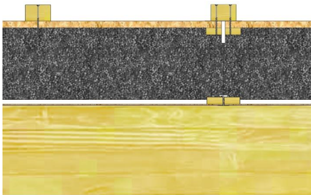
Figuur 9 - Bevestiging tengels door onderliggende verstijvers
